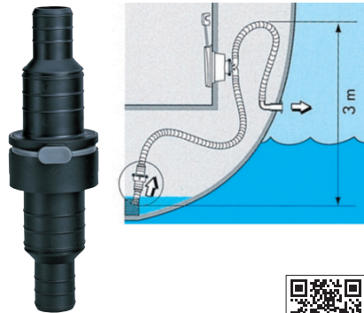
ノンリターンバルブ
